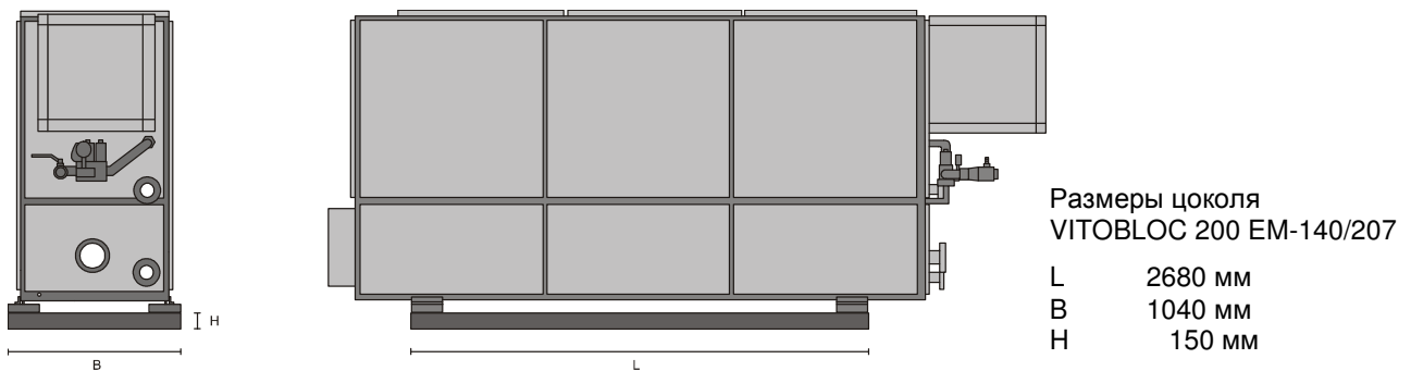
Рис.7 Размер цоколя
