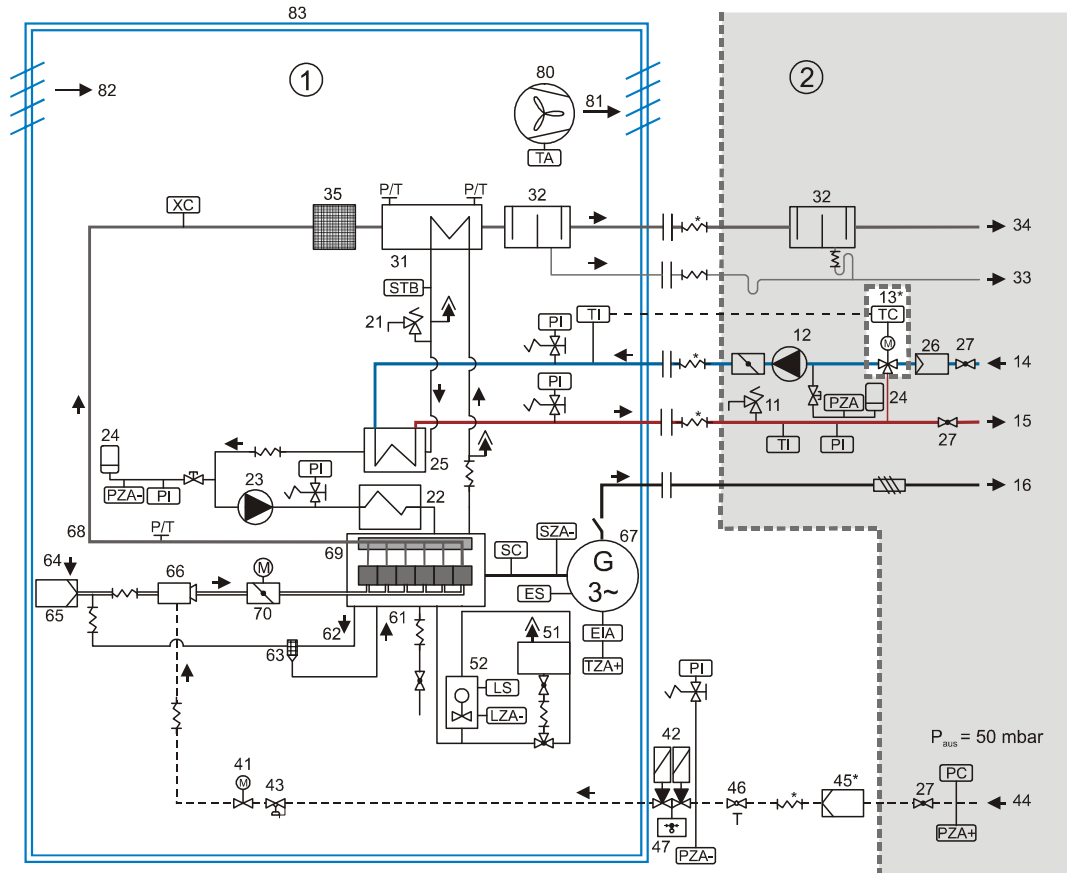
Рис.2 Устройства контроля
