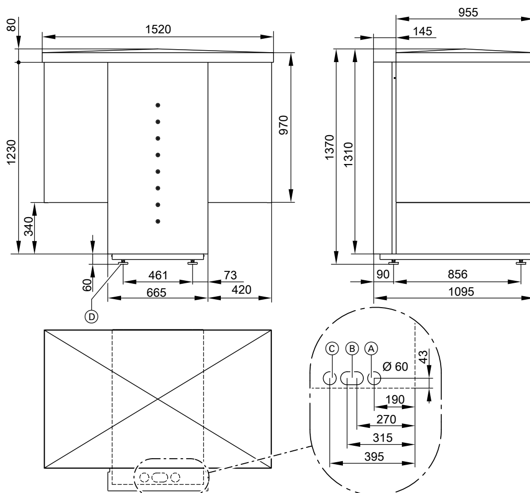
Тип AWO 110 и 114
