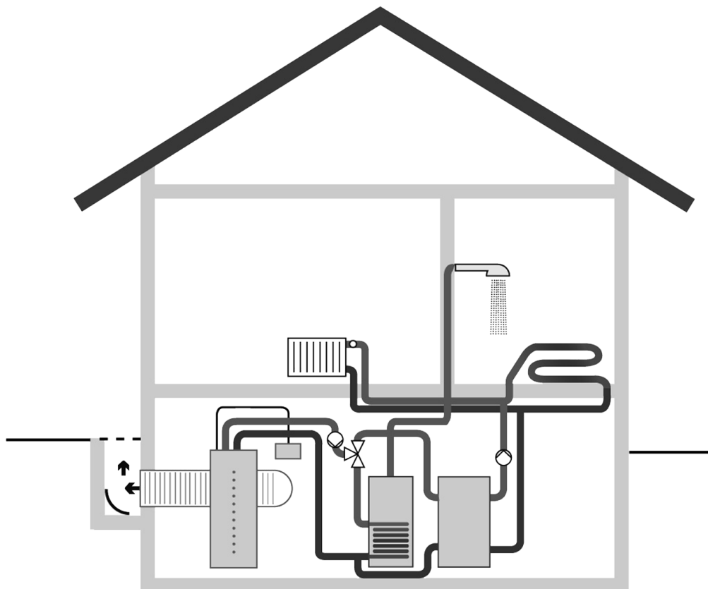
Vitocal 350-A, тип AWI – воздушно-водяной тепловой насос для установки в помещениях
